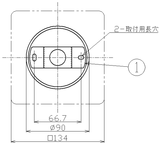
取付寸法 (㊤ 矢視)
