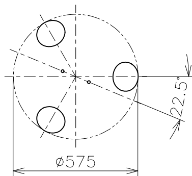
灯具配置 / 取付角度 (下面ヨリ)
