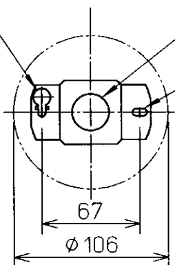
取付寸法(矢視a)
