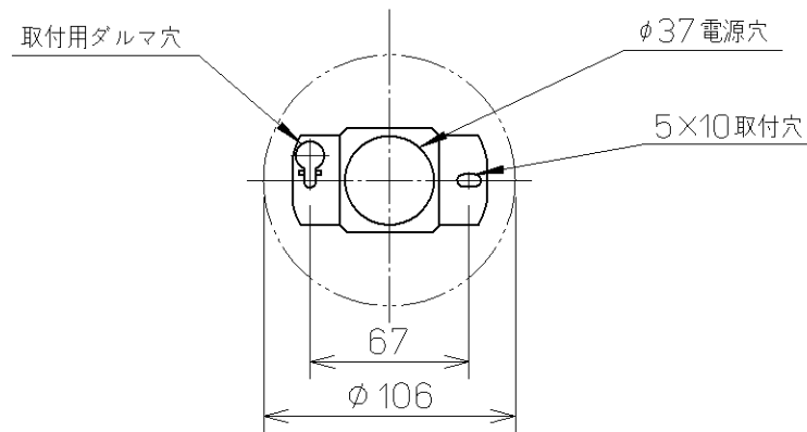
取付寸法 ( 矢視a )
