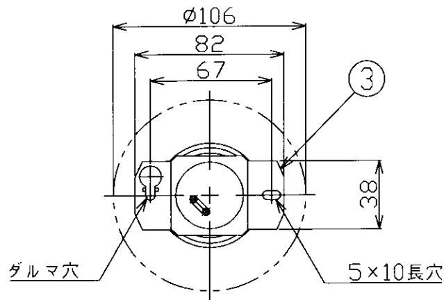
取付寸法（矢視②）
