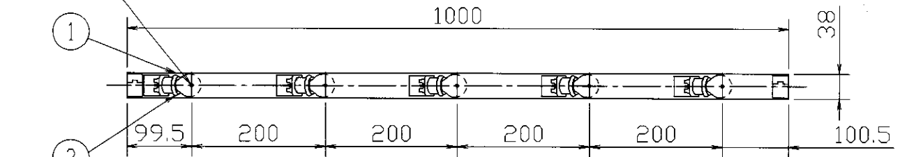
<施工最小寸法・壁付>
