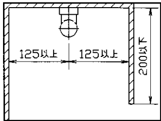
<施工最小寸法・直付>
