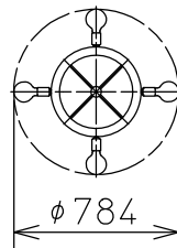
灯具配置図
