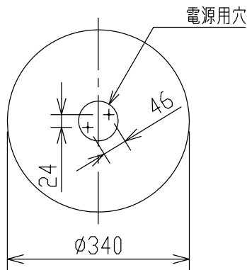
取付寸法(矢視 ②)
