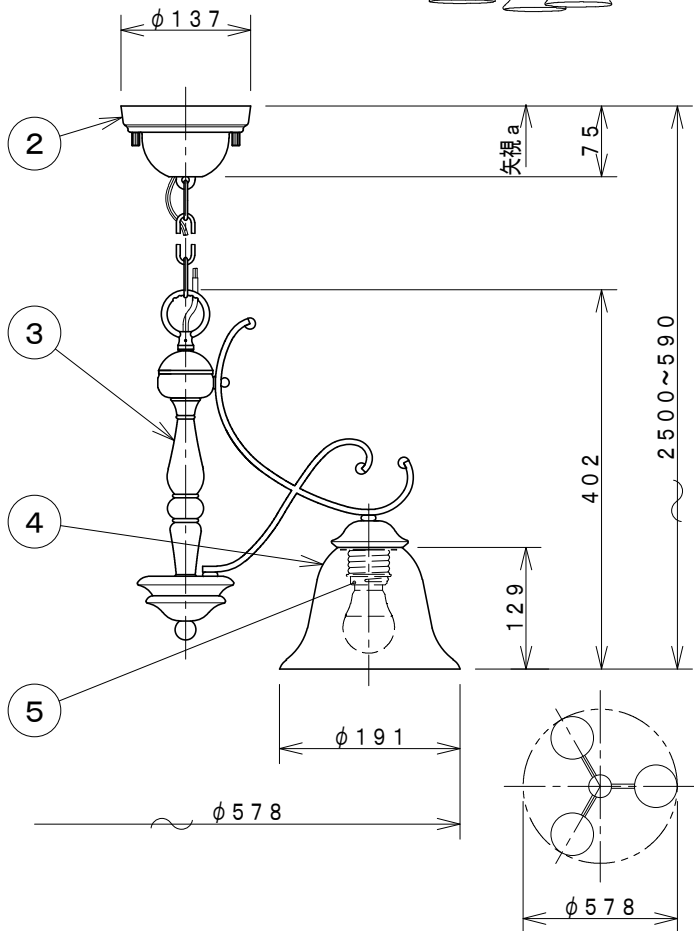
灯具配置図
