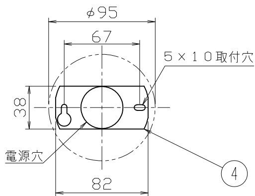
取付寸法（矢視 ④）
