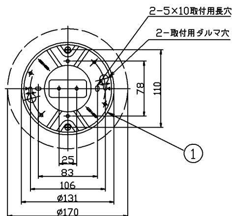
取付寸法 (a 矢視)
