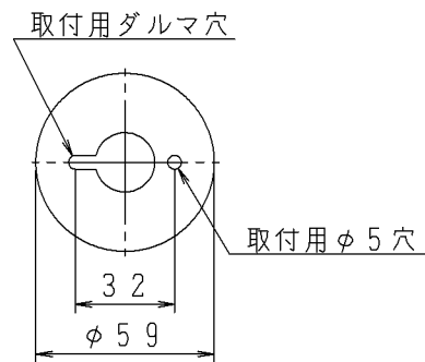
取付寸法（矢視①）
