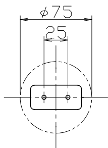
取付寸法（矢視 ①）
