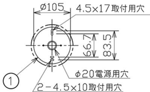
取付寸法 (矢視 a)
