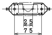
取付寸法(矢視⑨)
