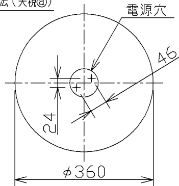
取付寸法（矢視②）
