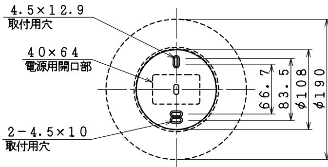
取付寸法(矢視 ⑧)
