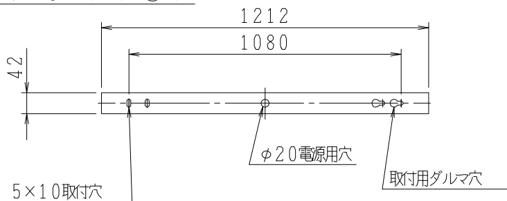
取付寸法（矢視 ③）
