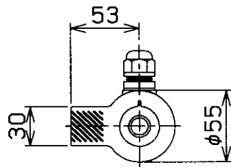
a 矢視図
