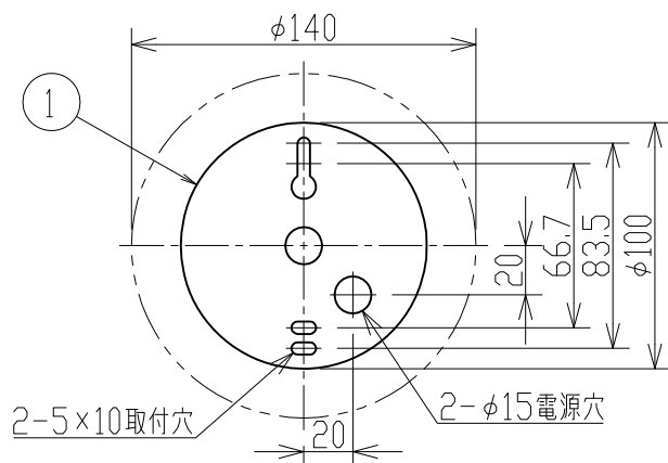
取付寸法(矢視a)
