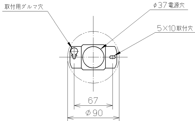
取付寸法（矢視a）
