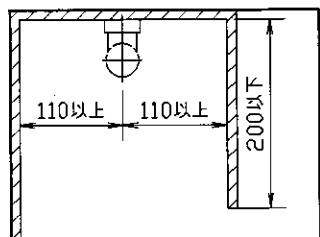
<施工最小寸法・直付>
