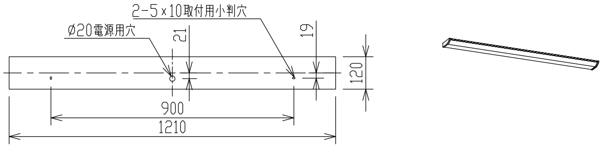
取付寸法(矢視 ㊸)
