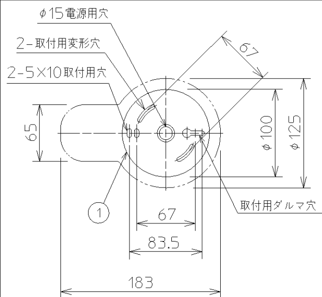
取付寸法（矢視a）
