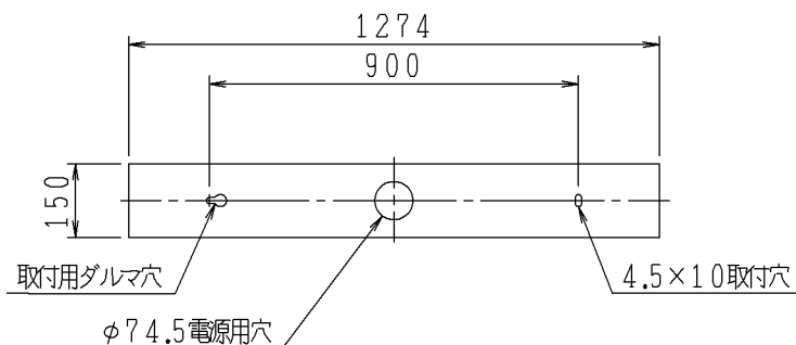
取付寸法（矢視 ㊸）
