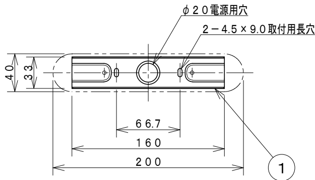
取付寸法 (矢視 a)
