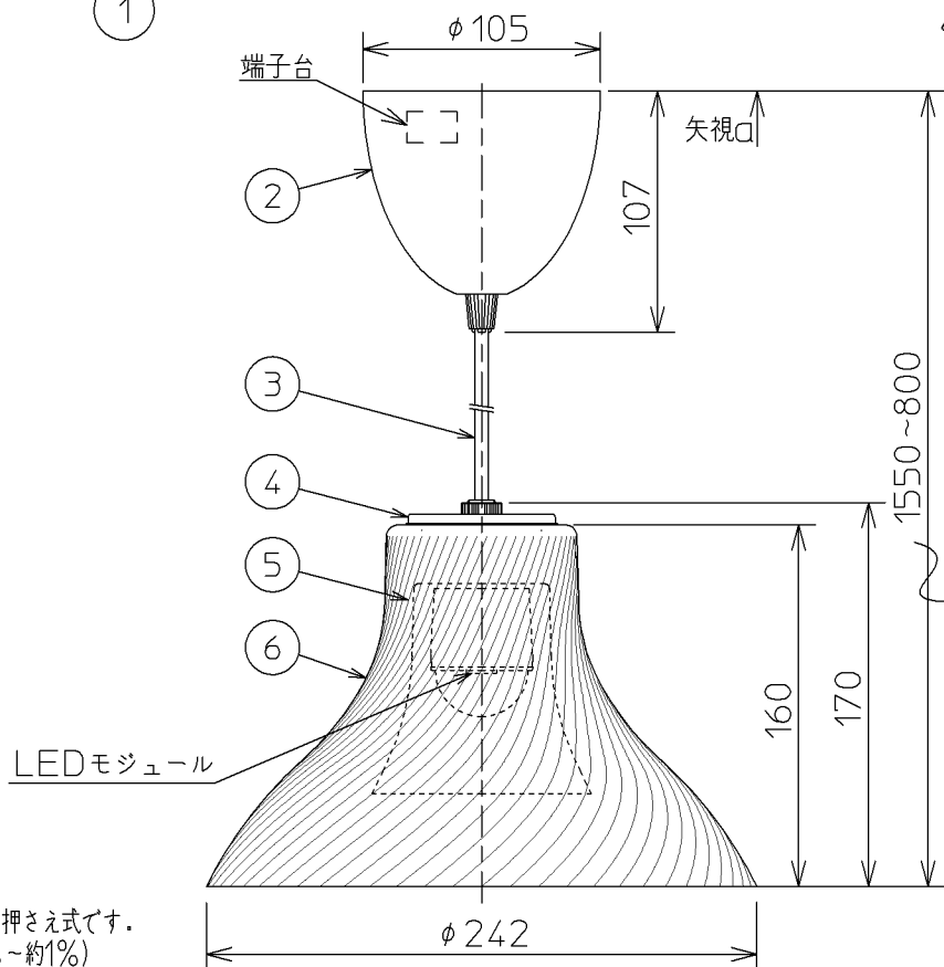
取付寸法（矢視a）
