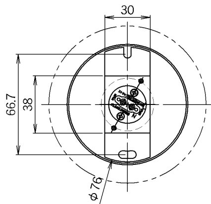
取付寸法 (矢視 ③)
