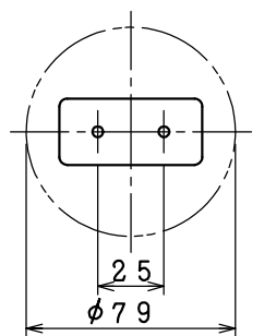
取付寸法(矢視 ②)
