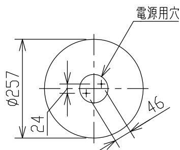
取付寸法(矢視 ㊟)
