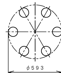
灯具配置図
