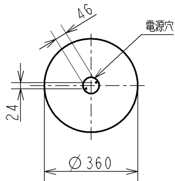
取付寸法（矢視 ㊤）
