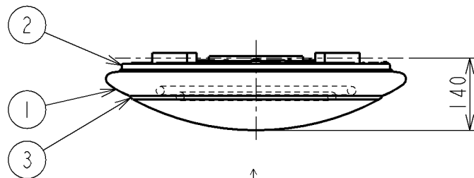
矢視 ㊦
