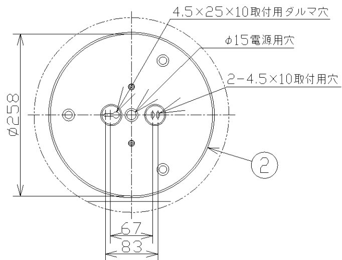
取付寸法 (矢視@)
