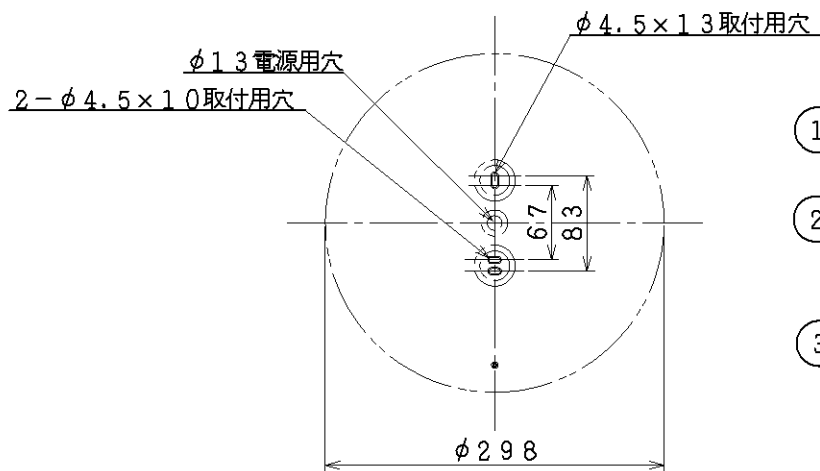
取付寸法 ( 矢視 (a) )
