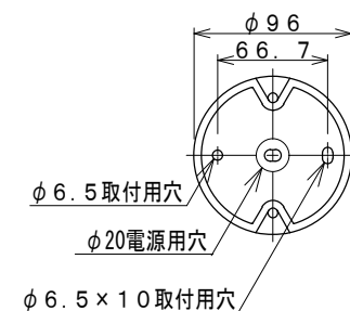
取付寸法(矢視@)
