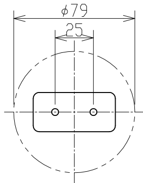
取付寸法(矢視a) (縮尺1/2.5)
