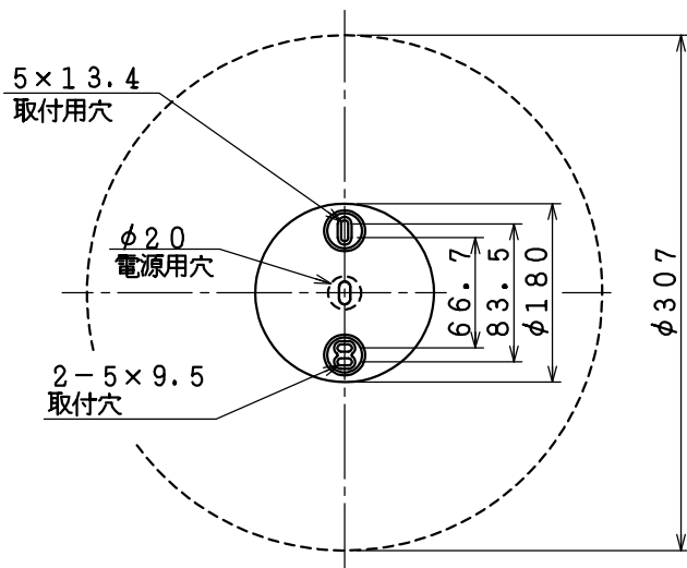
取付寸法（矢視①）
