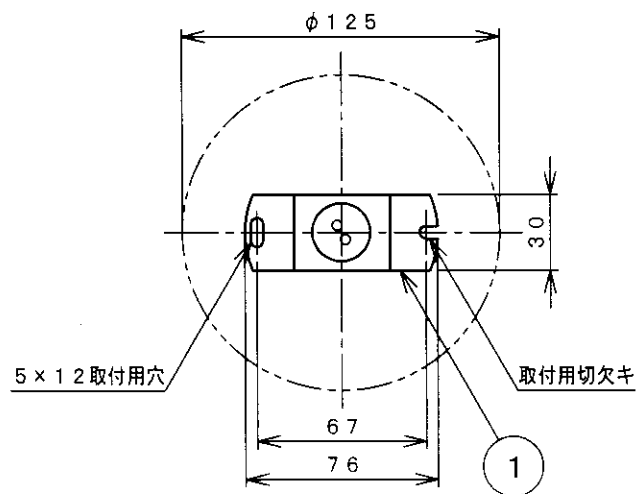
取付寸法（矢視 a）
