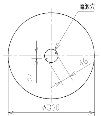
取付寸法 (矢視 ①)
