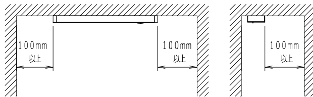
取付寸法 壁付の場合（矢視 ㊸）
