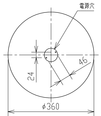
取付寸法（矢視 (a)）
