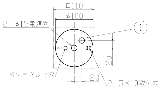
取付寸法 (矢視 ㊶)
