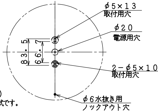
取付寸法(矢視①)
