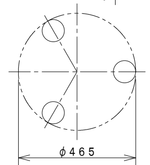
灯具配置図
