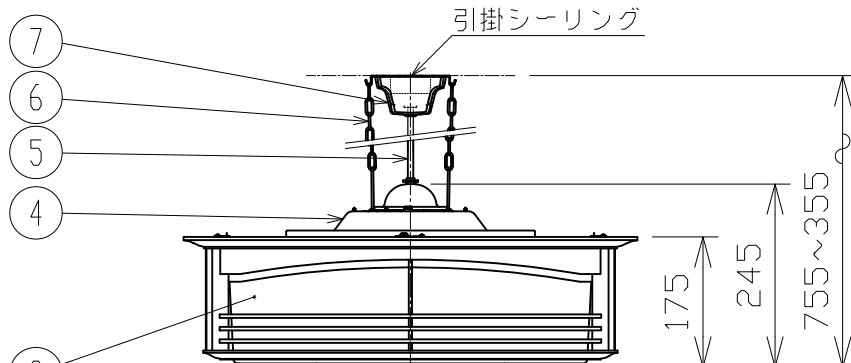
取付寸法（矢視 (a)）
