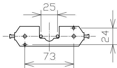
取付寸法（矢視 (a)）
