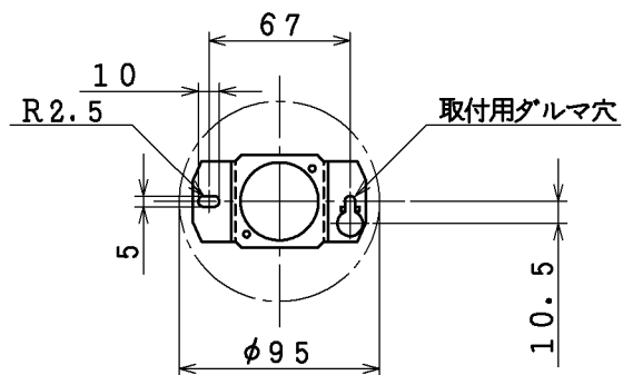
取付寸法(矢視 ㊸)
