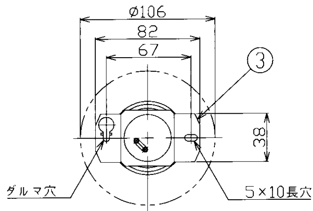
取付寸法（矢視④）
