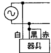
<単相 2 線 2 線引き・平常時消灯しない場合>
