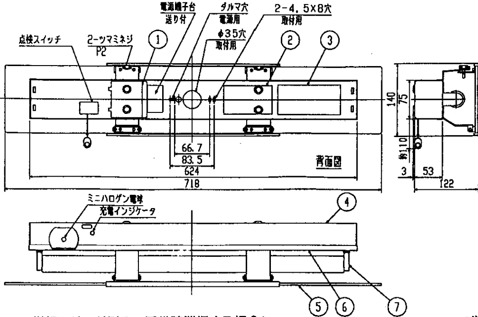
<単相 2 線 3 線引き・平常時消灯する場合>
