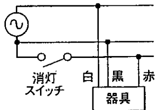
<単相 2 線 3 線引き・平常時消灯する場合>
