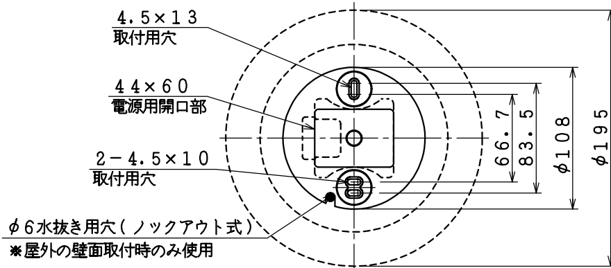
取付寸法(矢視 ⑧)
